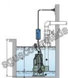
Bomba sumergible "Aguas Fangosas" 2 c.v. Mono Canal
